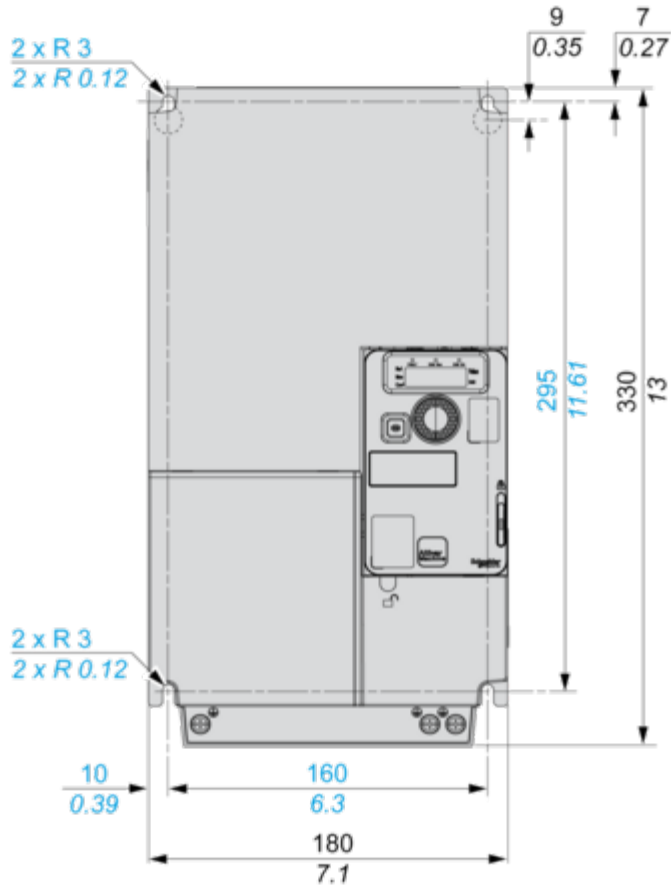
Vistas lateral derecha y frontal con placa CEM
