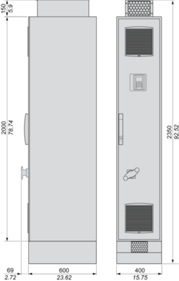
Vistas lateral derecha y frontal
