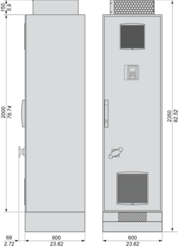
Vistas lateral derecha y frontal
